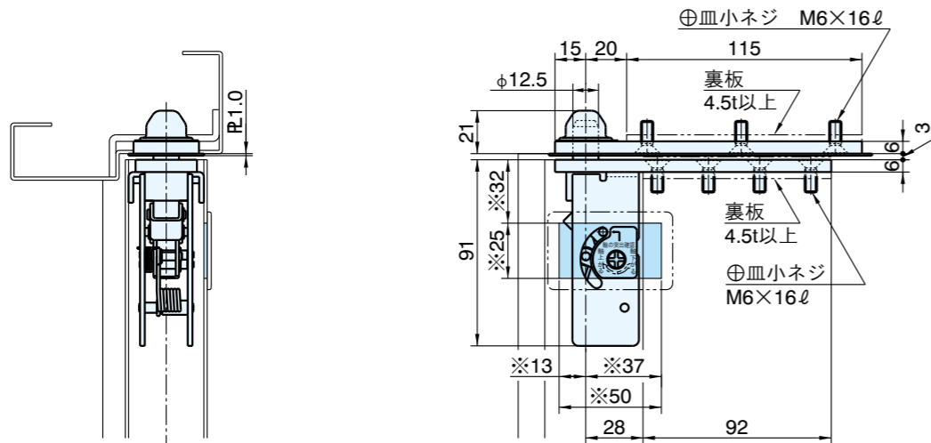
トップピボット(上枠側)
