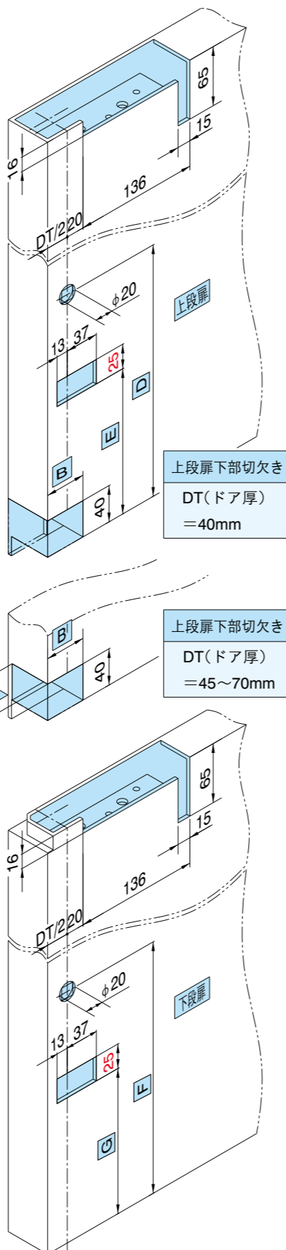
扉切欠き寸法図
