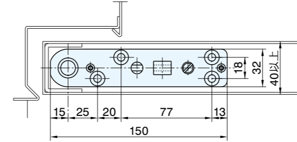
トップピボット(ドア側)
