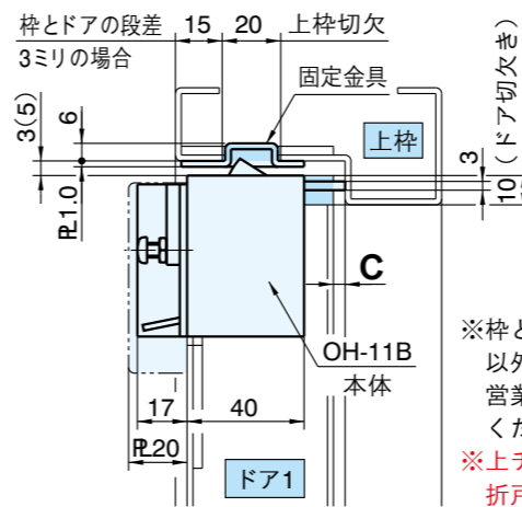
戸当り側ドア全閉時納り図
