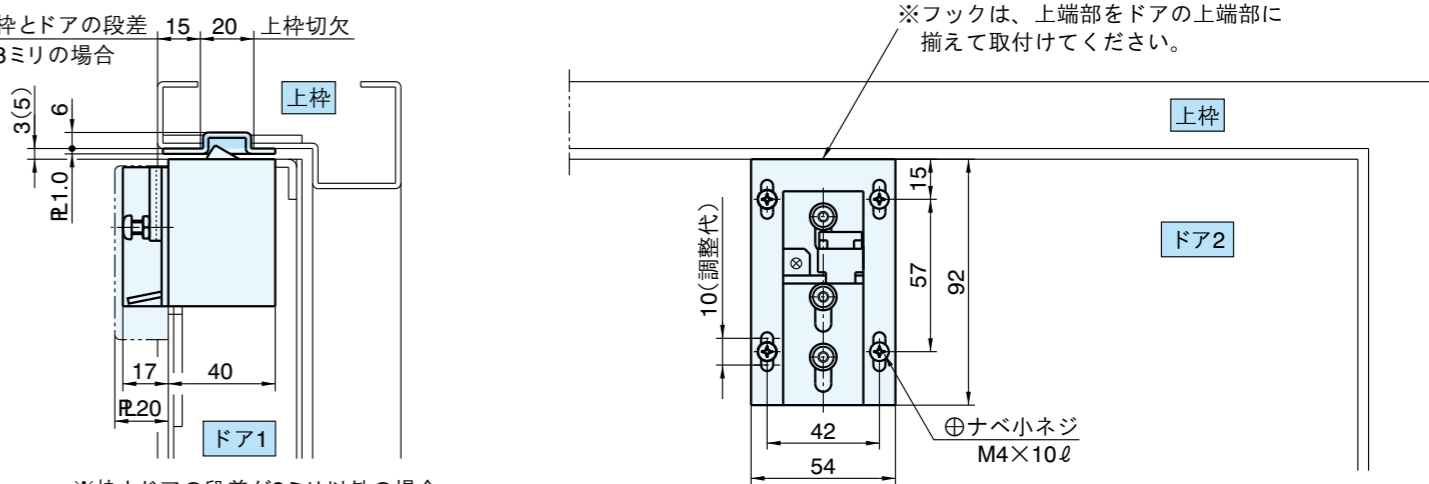
戸当り側ドア全閉時納り図
