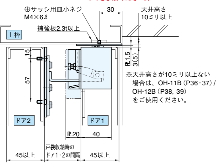
戸袋側ドア全開時納り図
