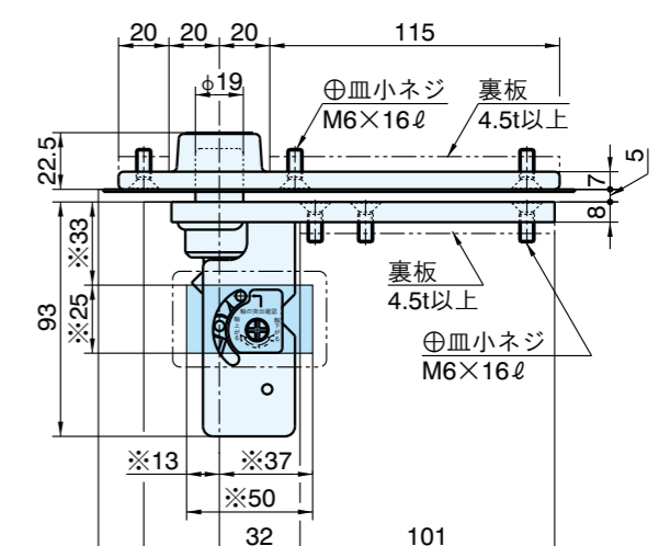
トップピボット(ドア側)
