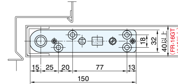
トップピボット(ドア側)
