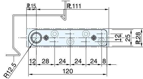
トップピボット(上枠側)
