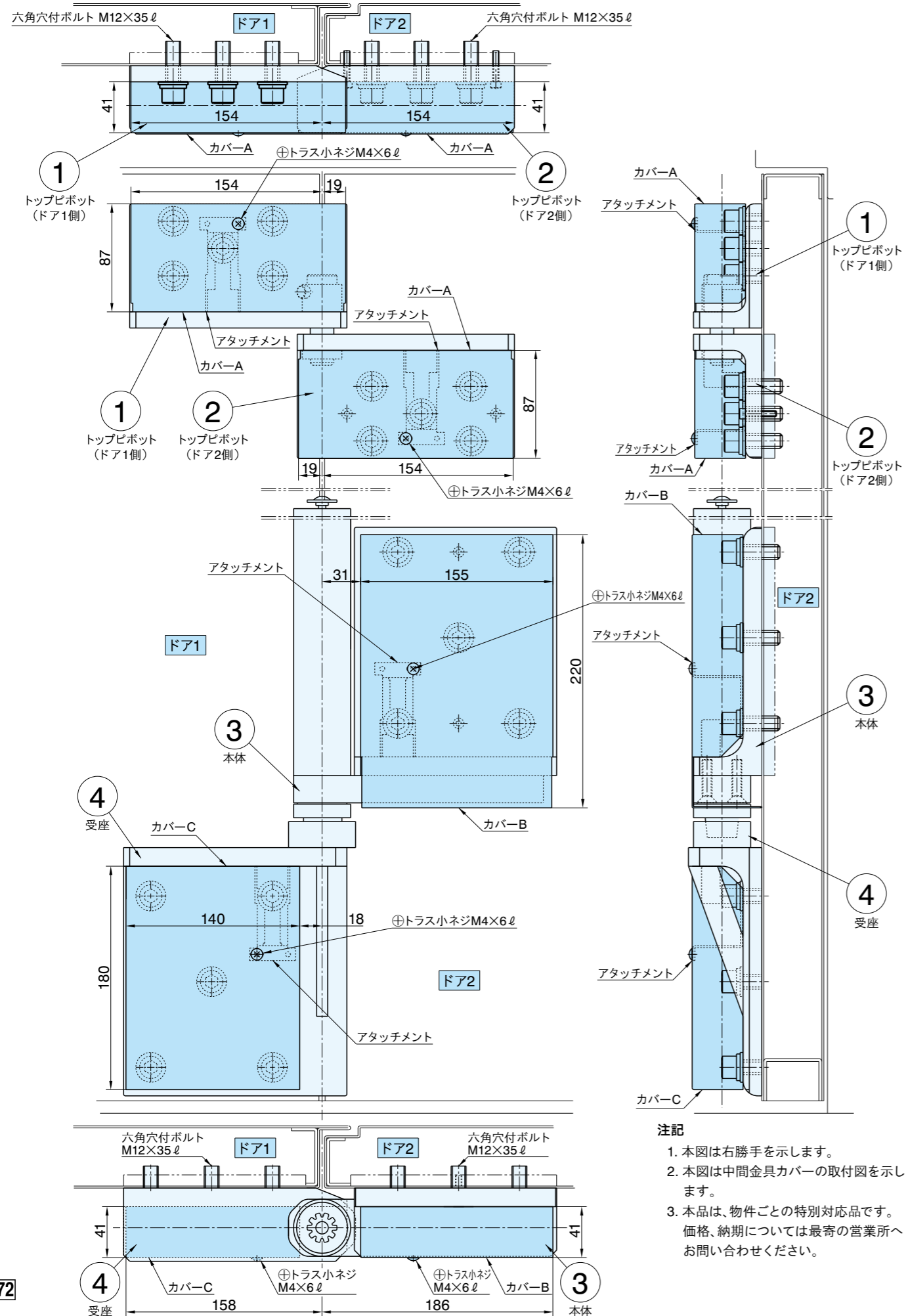
取付寸法図
