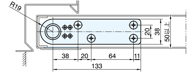
トップピボット(ドア側)
