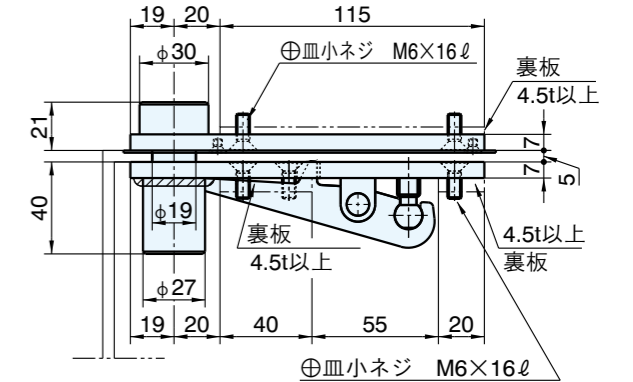
トップピボット(ドア側)
