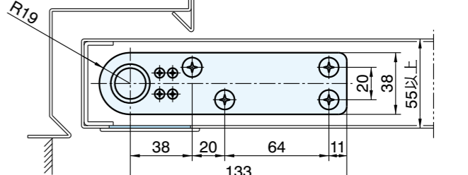
トップピボット(ドア側)
