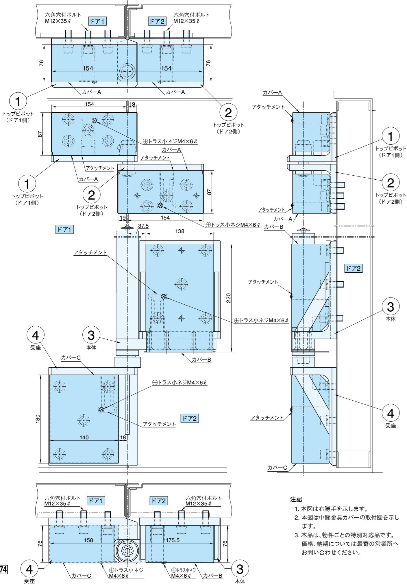
取付寸法図
