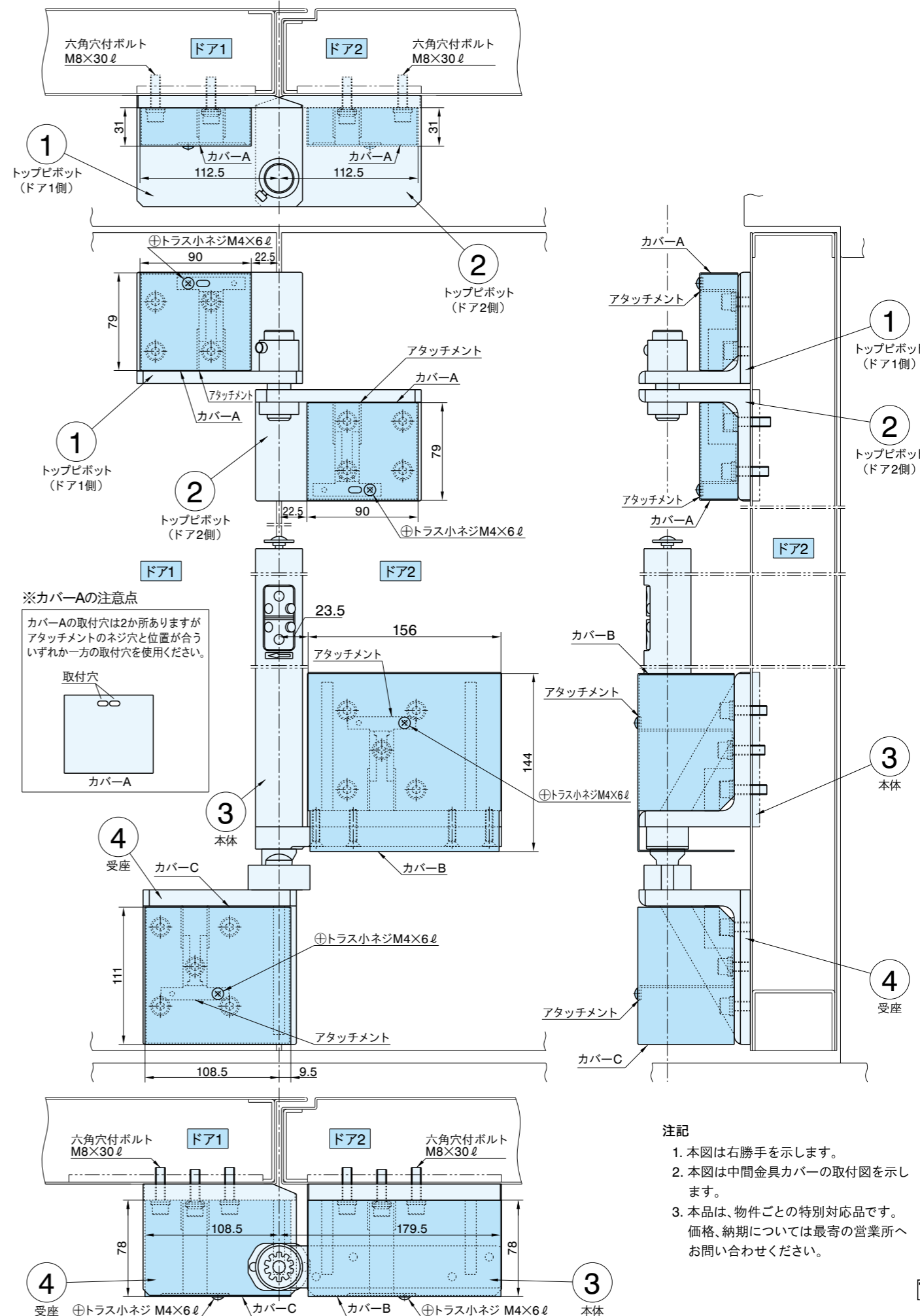
取付寸法図
