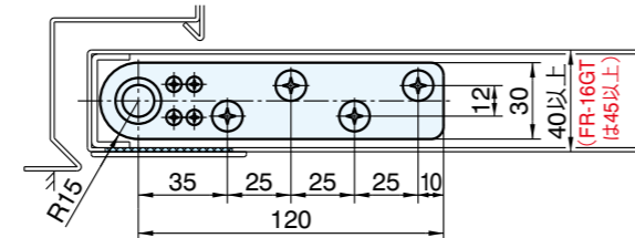
トップピボット(ドア側)
