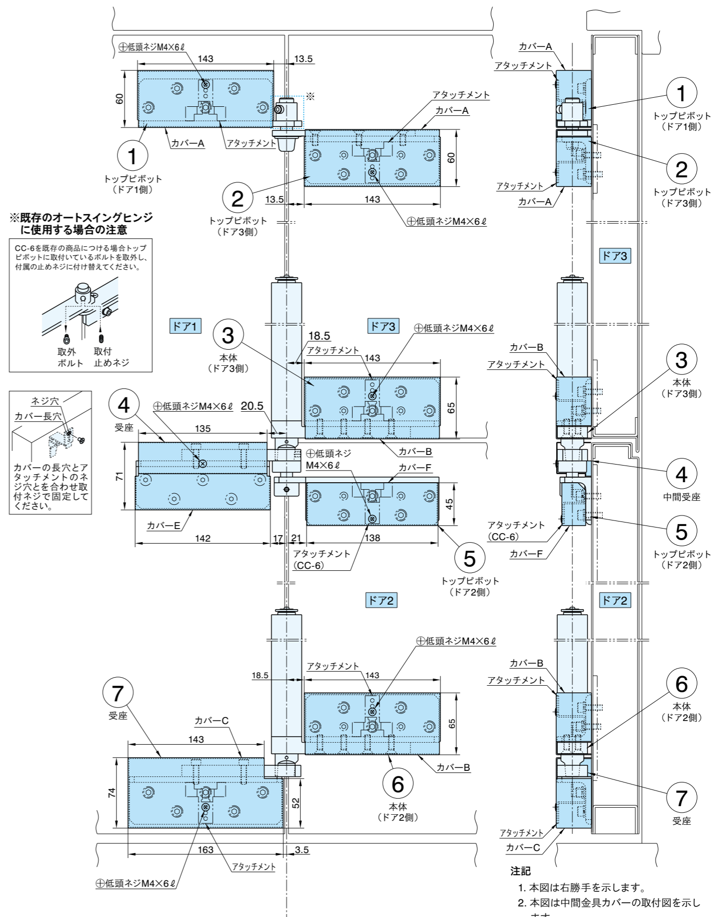
取付寸法図
