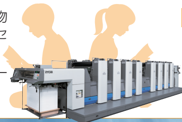
A全判オフセット8色印刷機 [RYOBI 928P]
