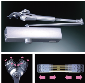
広範囲のネジ穴に対応できる取替用ドアクローザ
