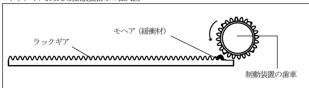
ラックギアおよび制動装置歯車の拡大図
